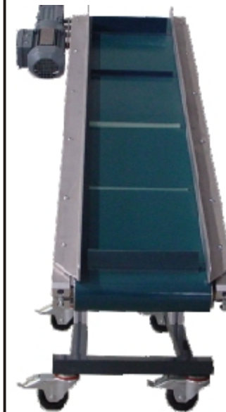
GF-80 zum Transport von Granulaten, Angüssen, Kartonagen sowie von Bauteilen mit Stückgewichten bis ca. 50 kg
